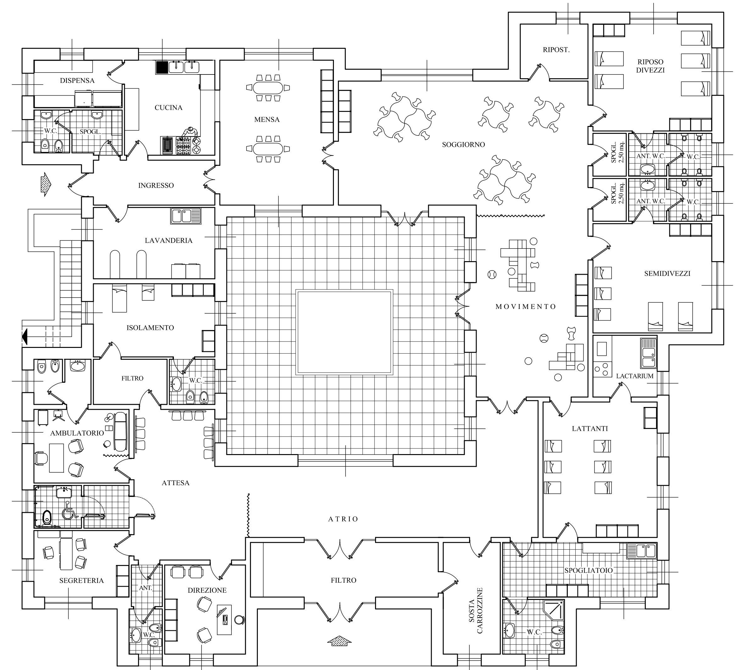
LEGAUT DEGLI ARREDI scala 1:100
